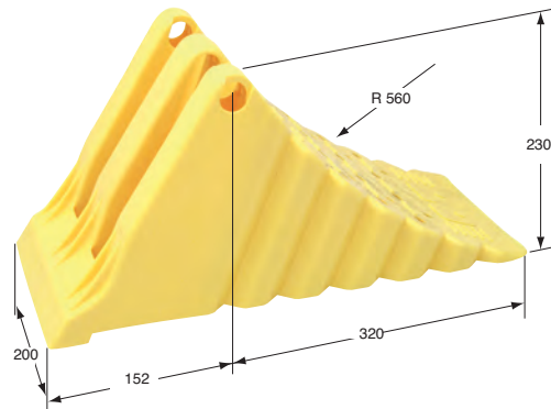
39.51300 \frac{Kg}{Kg} 1,875 Calço para rodas NG 53 (DIN 76051-11/92) Raio máximo do pneu = 560 mm
