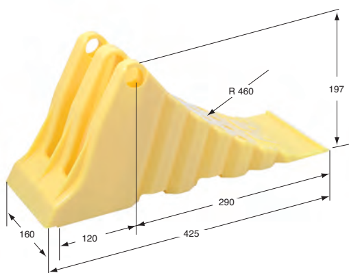
39.51298 \frac{Kg}{Kg} 1,100 Calço para rodas NG 46 (DIN 76051-11/92) Raio máximo do pneu = 460 mm
